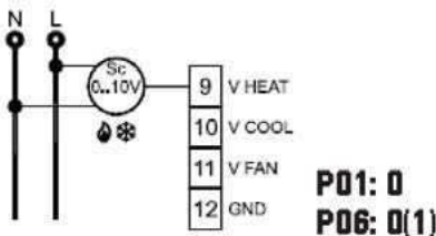
Sistema a 2 tubos con servovolt 0...10V.
