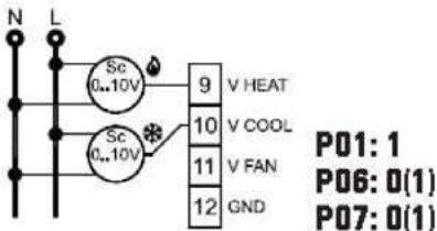
Sistema a 4 tubos con dos servocontroles 0...10V.
