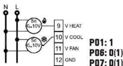
Sistema a 4 tubos con dos servovalvulas 0...10V.
