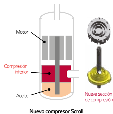
Nuevo compresor Scroll
