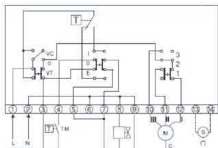
Válvula calor y frío
