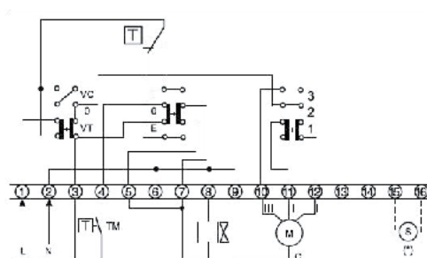
Válvula calor y frío
