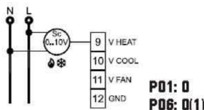
Sistema a 2 tubos con servovalvula 0...10V.
