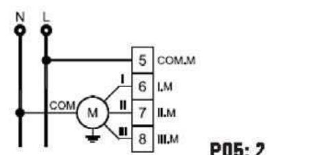
Conexión de un ventilador con motor de tres velocidades.
