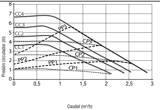
Presión residual disponible en instalación para CONNECT 3D LE y CONNECT 2D LE
