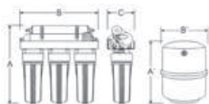
Dimensiones (mm)
